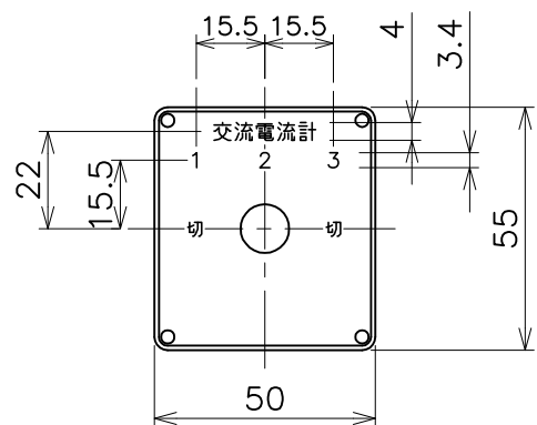
铭板文字記入位置図 (N-1:材質=アルミ製)
