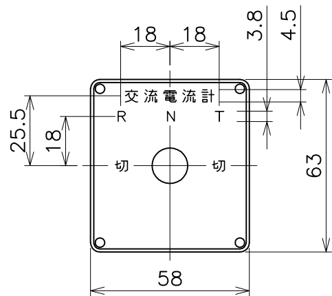
铭板文字記入位置図 (N-31:材質=アルミ製)
