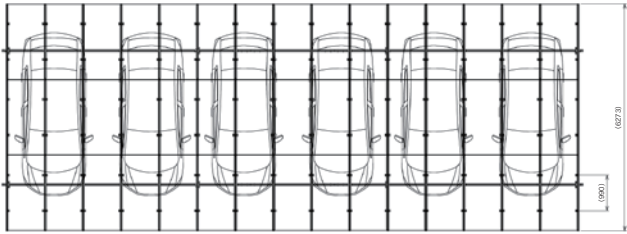
平面図 SCALE 1:100
