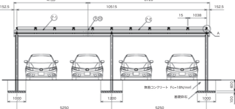
正面図 SCALE 1:100
