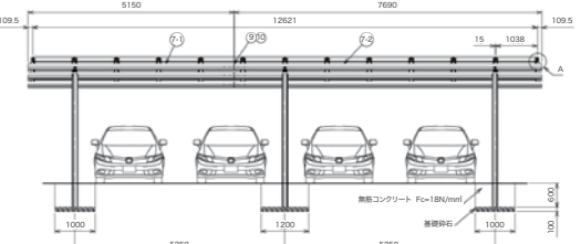
正面図 SCALE 1:100
