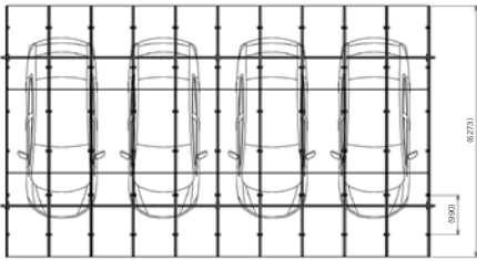
平面図 SCALE 1:100
