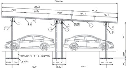
側面図 SCALE 1:100
