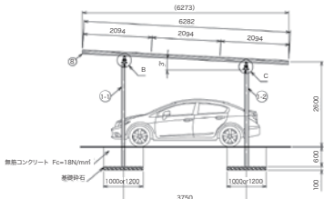
側面図 SCALE 1:100
