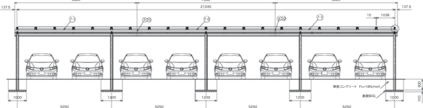
正面図 SCALE 1:100
