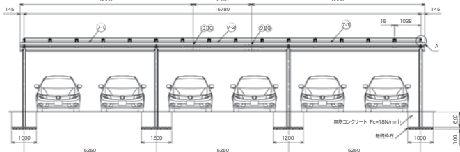
正面図 SCALE 1:100
