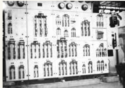
昭和8年 九州大学納入低圧動力大理石盤
